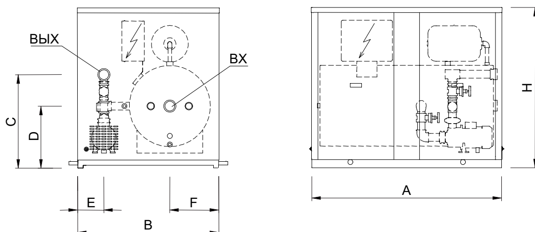
Размеры горизонтальных НРТ
