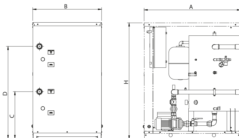
Размеры вертикальных НРТ
